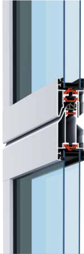
Perfil térmico, 42 mm
