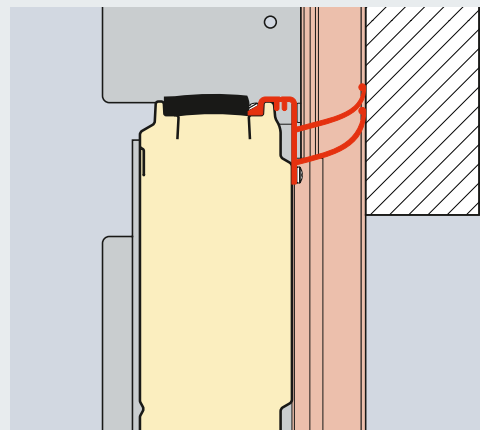
Topo de dintel con ThermoFrame
